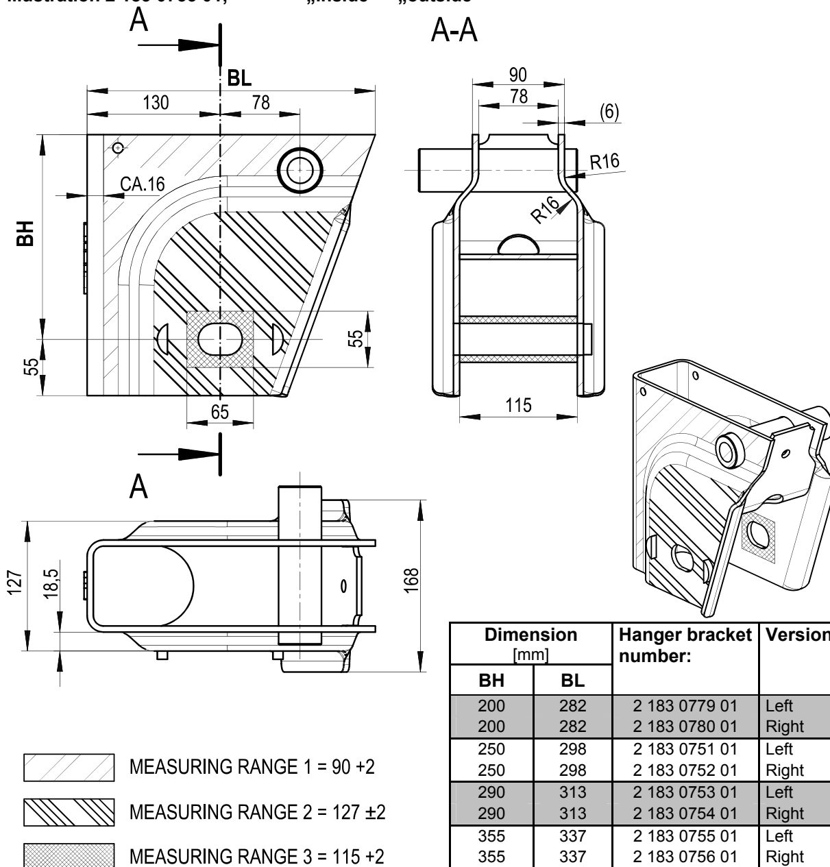
illustration 2 183 0753 01, „inside“ – „outside“
