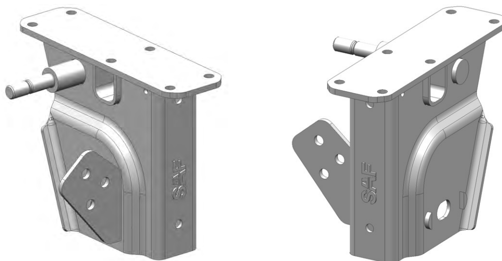
illustration 2 183 0879 00, „inside“ – „outside“
