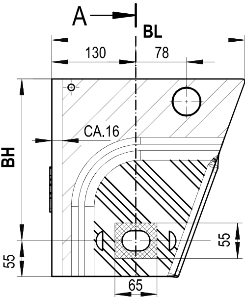
illustration 2 183 0747 01, „inside“ – „outside“
